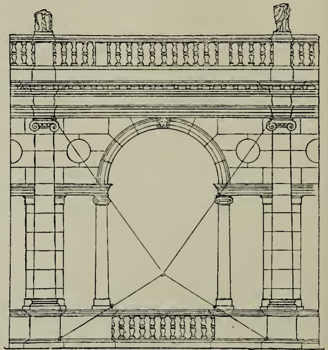
Abb. 81. Von der Basilica zu Vicenza. (Nach A. Thiersch im Handb. d. Archit.)
